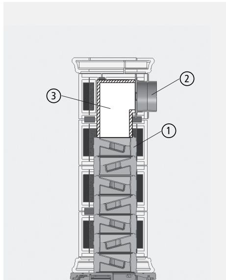
Abb. 3.5 Abgang hinten
