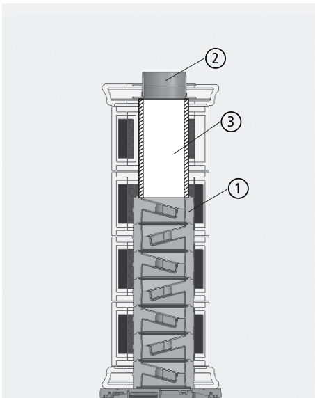
Abb. 3.4 Abgang oben
