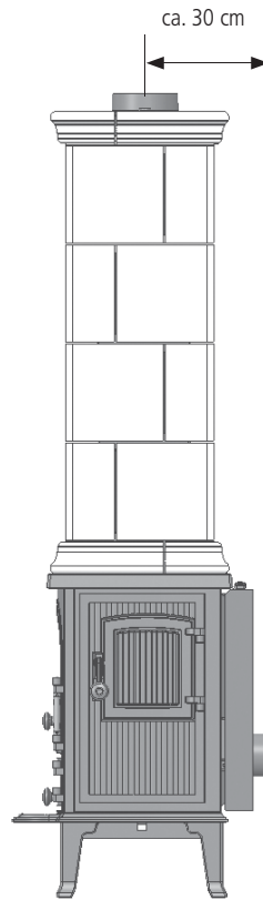
Abb. 3.9 Abgasanschluss nach oben
