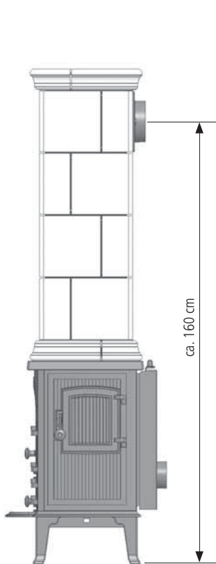
Abb. 3.8 Abgasanschluss nach hinten
