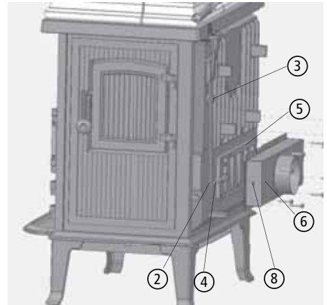
Abb. 3.7 Außenluftanschlusskasten montieren
