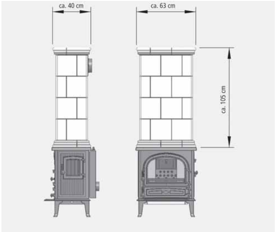
Abb. 10.1 Abmessungen der Ofenverkleidung
