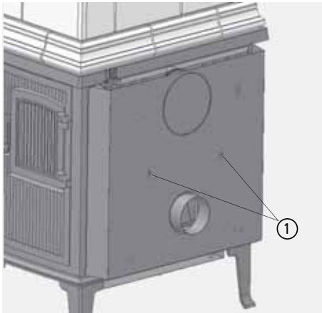
Abb. 3.6 Rückwand-Strahlungsblech demontieren
