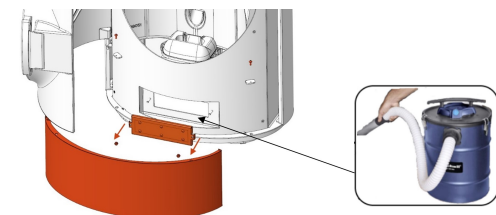
Abb. 36: Rauchgasbereich aussaugen
