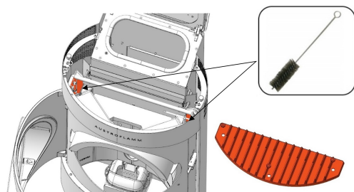
Abb. 35: Rauchgaszüge bürsten
