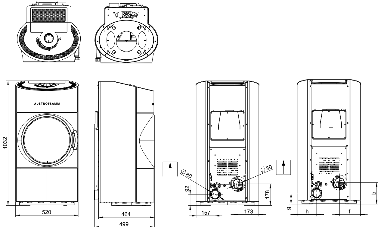
Abb. 3: Abmessungen Clou Compact Pellet
