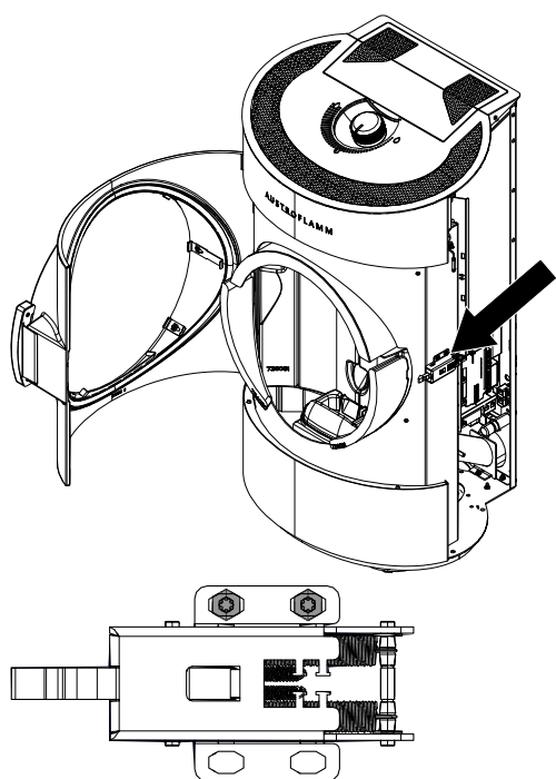
Abb. 23: Türverschluss einstellen
