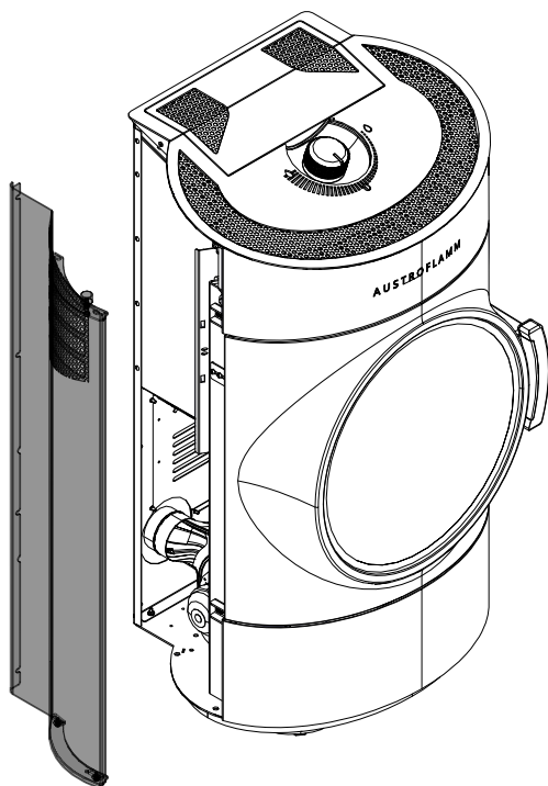
Abb. 20: Seitenverkleidung abnehmen
