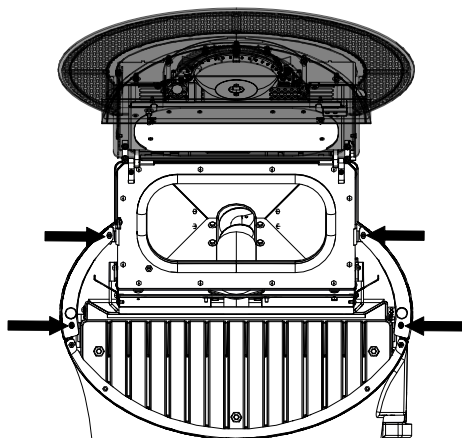
Abb. 43: Schrauben lösen
