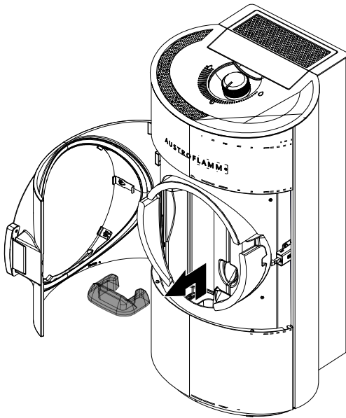
Abb. 27: Keramott-Stein entfernen
