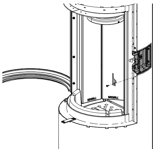
Abb. 41: Türeingriff montieren
