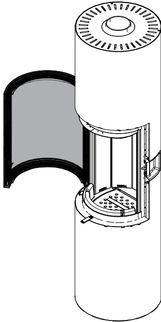
Abb. 42: Tür öffnen
