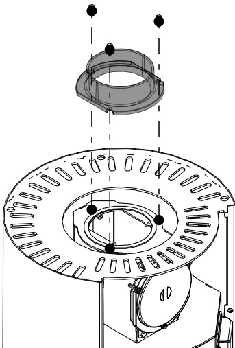
Abb. 19: Rauchrohrstutzen abmontieren
