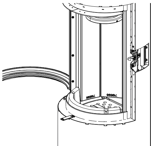
Abb. 40: Türverschluss einstellen
