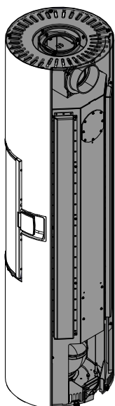
Abb. 56: Rückwand und Deckel wieder montieren
