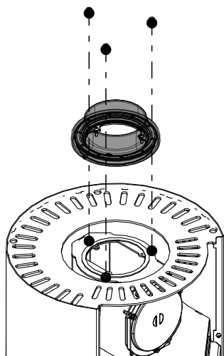
Abb. 20: Drehrauchrohrstutzen montieren
