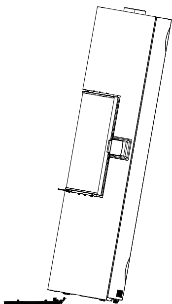
Abb. 20: Drehrauchrohrstutzen montieren
