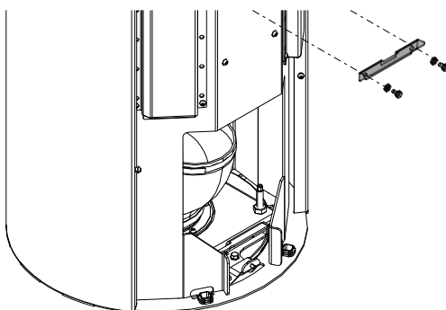
Abb. 31: HMS-Halter montieren
