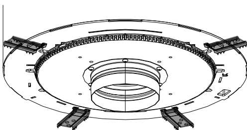
Abb. 8: Transportsicherung entfernen
