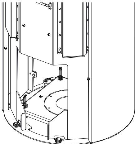
Abb. 35: Kaminofen ausrichten
