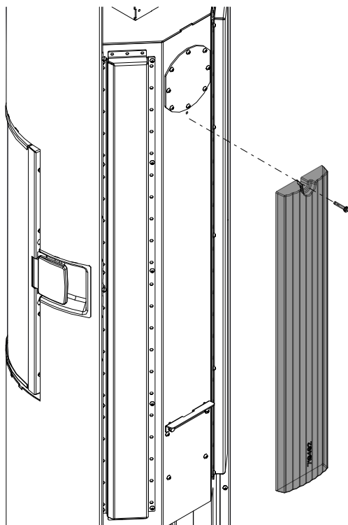
Abb. 32: HMS-Stein montieren
