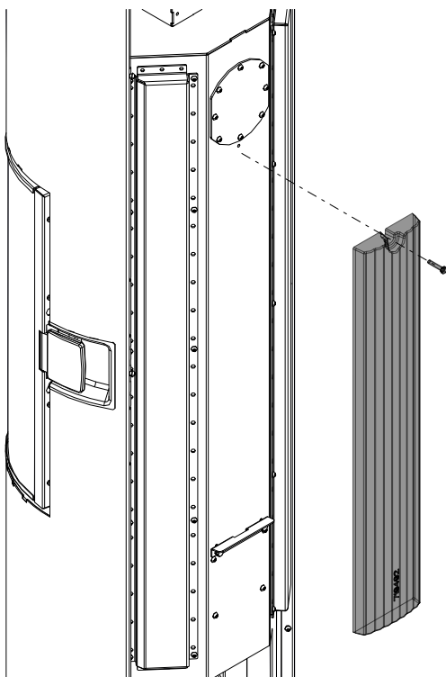
Abb. 55: HMS-Stein demontieren
