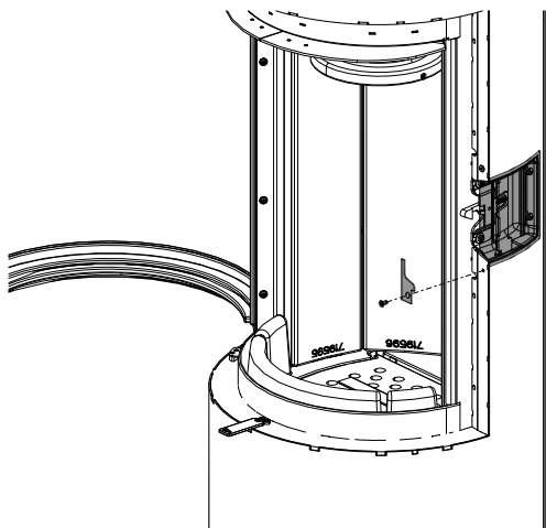
Abb. 39: Türeingriff demontieren
