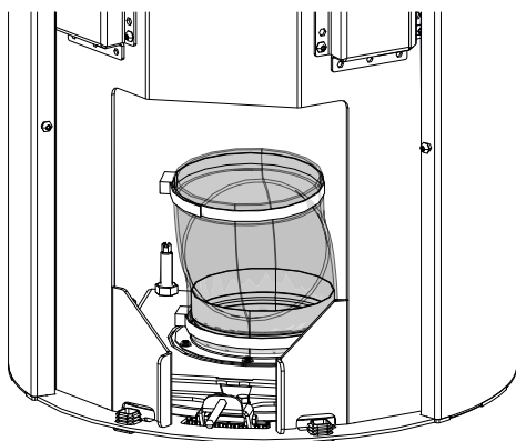
Abb. 27: Rohr befestigen
