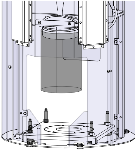
Abb. 17: Aluflexrohr befestigen.
