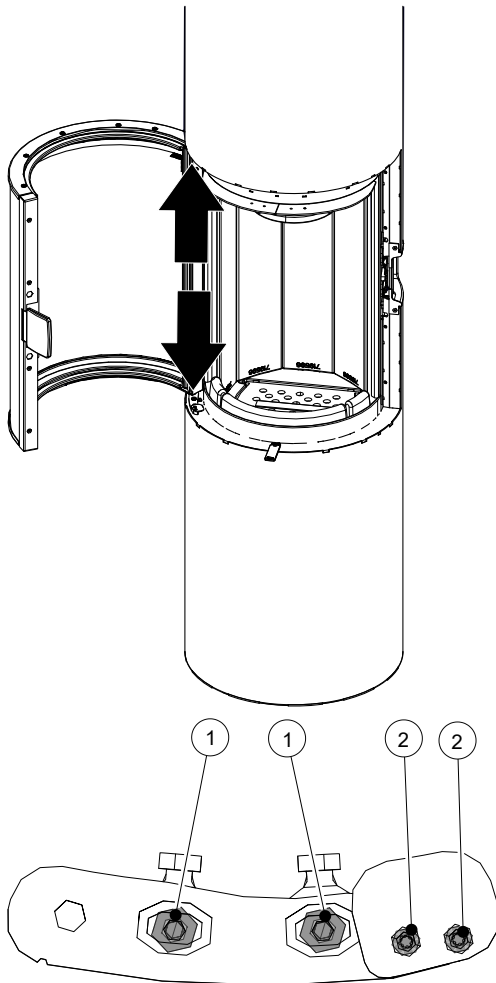
Abb. 37: Türeinstellschrauben
