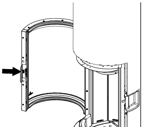
Abb. 43: Türschließkraft einstellen
