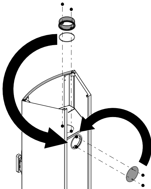
Abb. 10: Abdeckung und Stutzen tauschen
