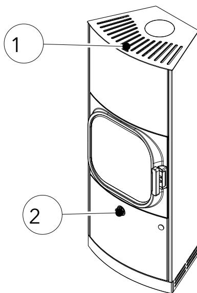
Abb. 23: Primär-Sekundärluftregler
