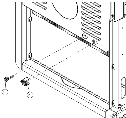
Abb. 18: Gleichstrombuchse u. Netzbuchse montieren
