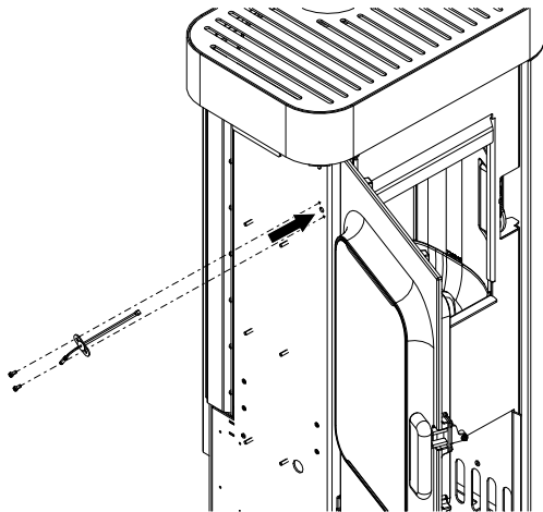
Abb. 17: Feuerraumtemperaturfühler befestigen
