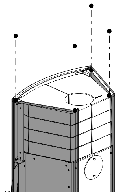
Abb. 34: Seitenverkleidung abnehmen
