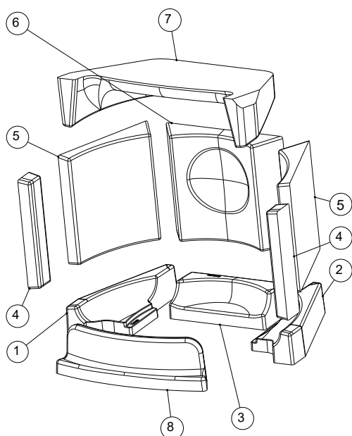
Abb. 13: Keramott montieren
