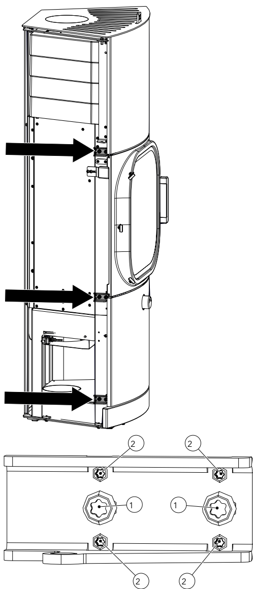
Abb. 20: Türeinstellschrauben
