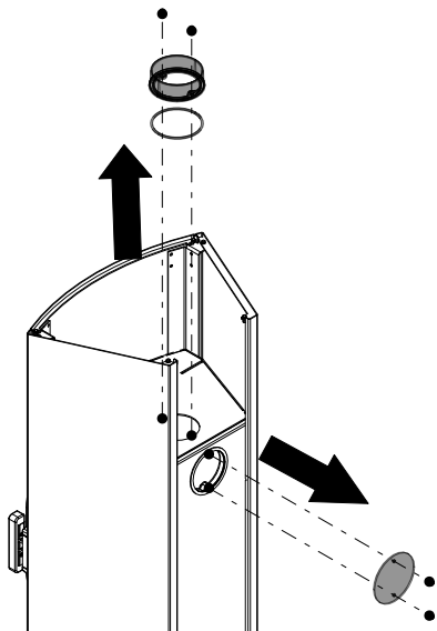
Abb. 9: Abdeckung und Rauchrohrstutzen demontieren
