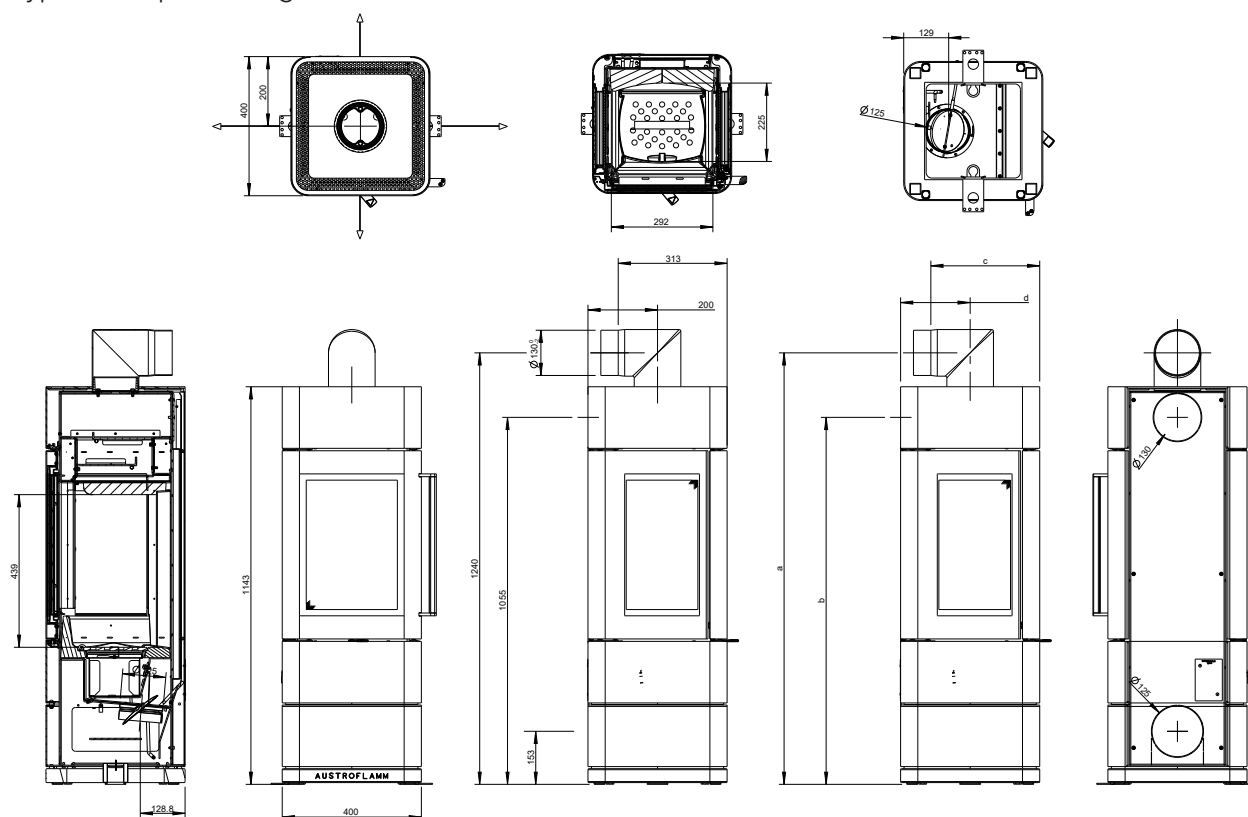
Abb. 2: Abmessungen
