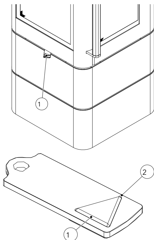
Abb. 32: Primär- Sekundärluftregler
