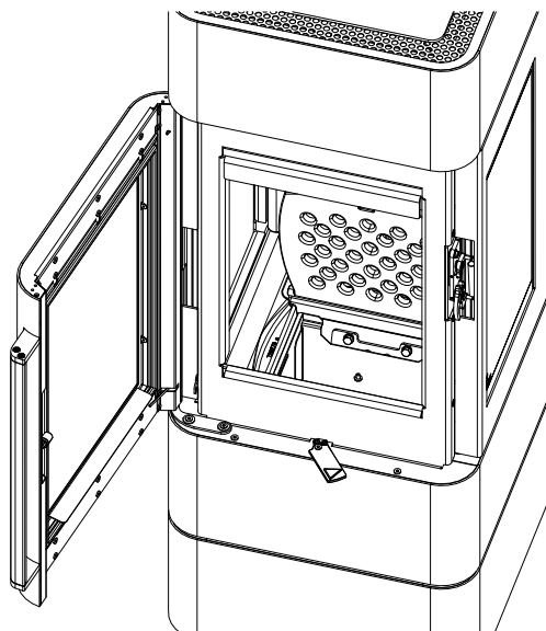
Abb. 35: Rost hochklappen
