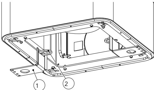
Abb. 7: Transportsicherung
