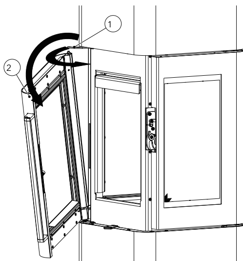
Abb. 42: Tür aushängen
