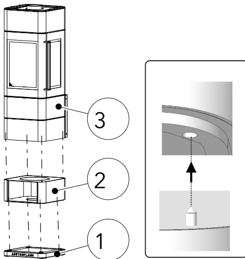
Abb. 16: Sockel montieren
