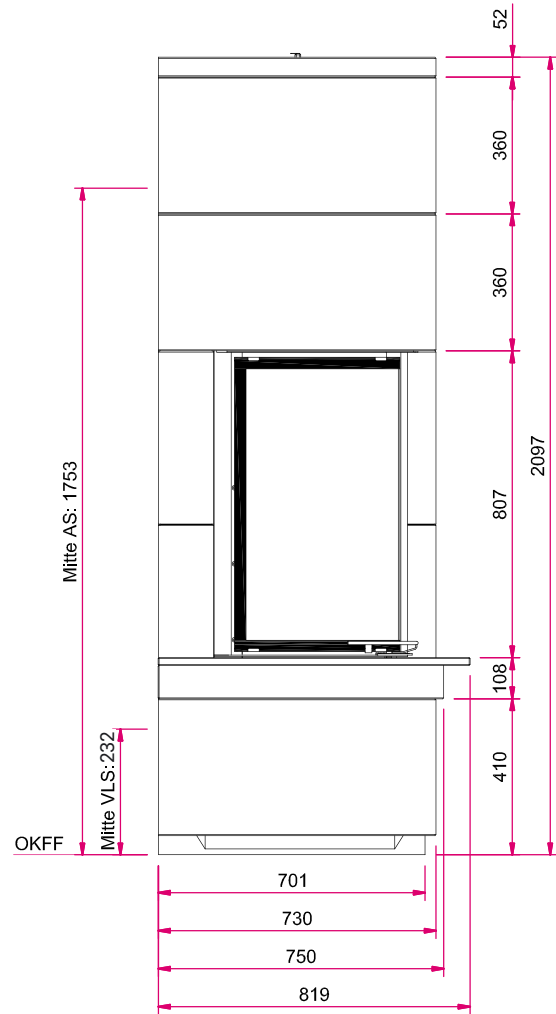
Seitenansicht
