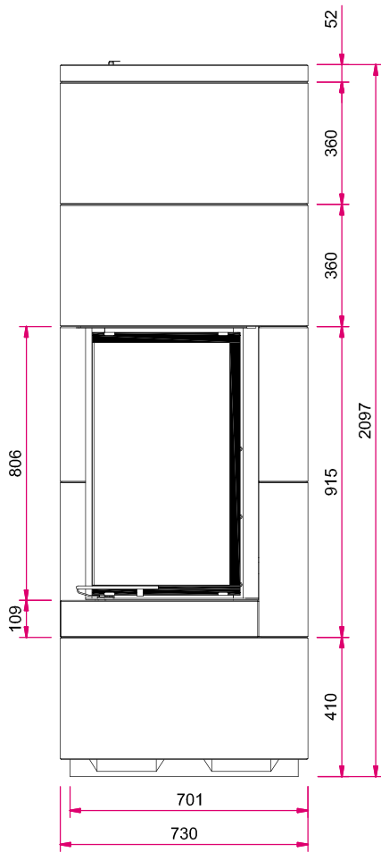
Frontansicht
