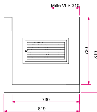
Draufsicht
