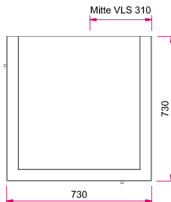
Draufsicht
