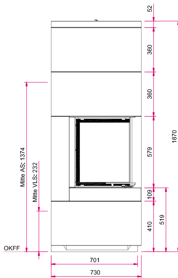
Seitenansicht
