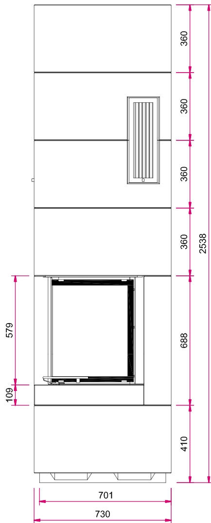
Frontansicht
