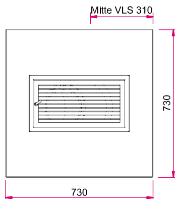
Draufsicht
