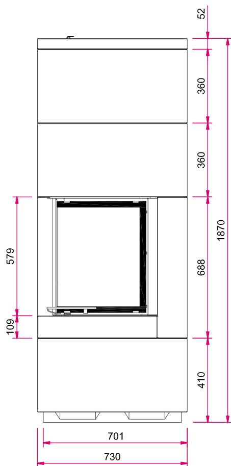
Frontansicht
