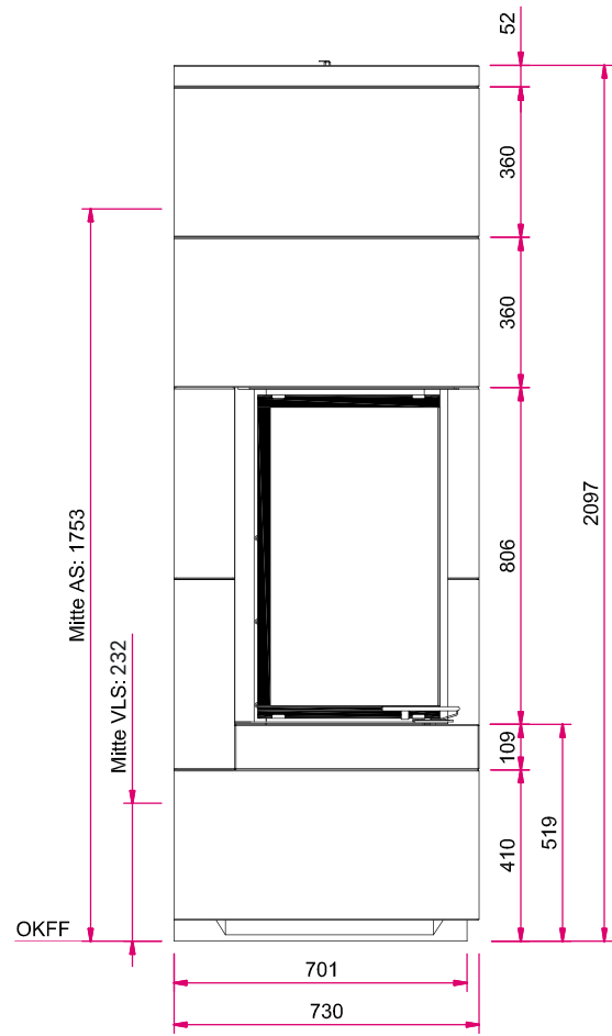
Seitenansicht
