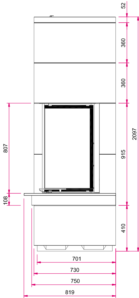
Frontansicht
