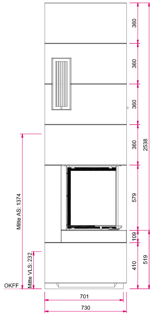
Seitenansicht
