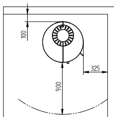
Avstånd til brännbar vägg med isolerad skorsten
