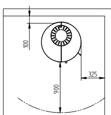
Avstånd til brännbar vägg Utan isolerad skorsten
