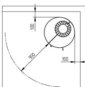
Afstand til brandbart uden isoleret røgrør
