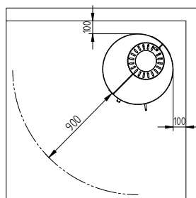
Afstand til brandbart med isoleret røgrør
