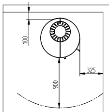
Abstand zu brennbarem Material ohne isoliertem Rauchrohr
