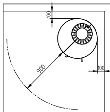
Abstand zu brennbarem Material ohne isoliertem Rauchrohr
