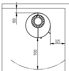
Avstand til brennbart uten isolerte røykrør
