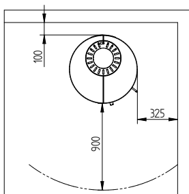
Afstand til brandbart med isoleret røgrør
