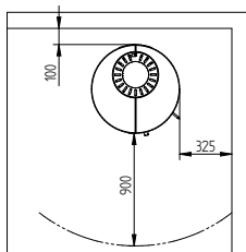
Abstand zu brennbarem Material mit isoliertem Rauchrohr
