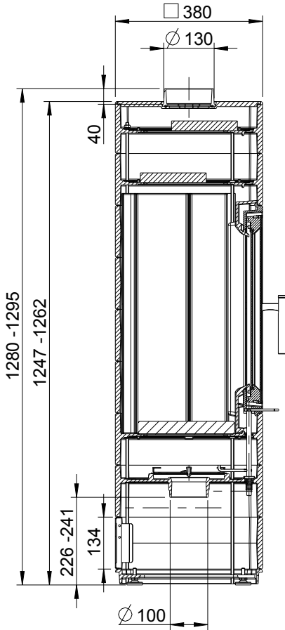
Abb. 3.11 Abgasanschluss, Maße bei Anschlussstutzen nach oben
