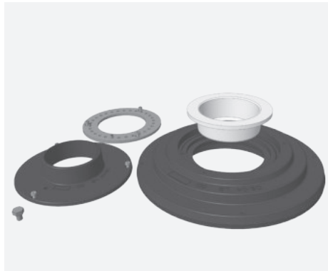
Abb. 3.7 Verbrennungsluftstutzen der Drehkonsole
