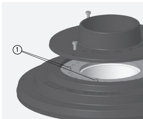
Abb. 3.8 Madenschrauben zur Einstellung des Drehwinkels
