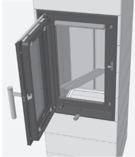
Abb. 4.13 Entnehmen des Bodenblechs im Brennraum
