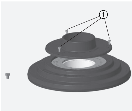
Abb. 3.5 Abnehmen des Konsolenoberteils
