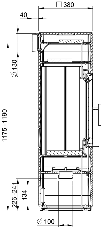
Abb. 3.12 Abgasanschluss, Maße bei Anschlussstutzen nach hinten
