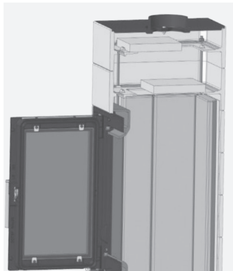
Abb. 4.14 Entnehmen des Bodenblechs im Brennraum
