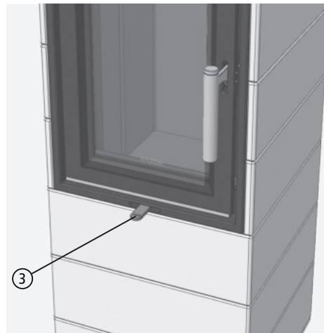
Abb. 4.2 Verbrennungslufthebel
