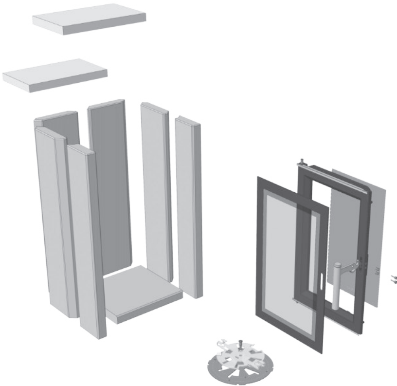
Abb. 8.1 Ersatzteilübersicht für CORNA
